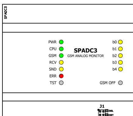
Obrázek 40 – Umístění switch J1
