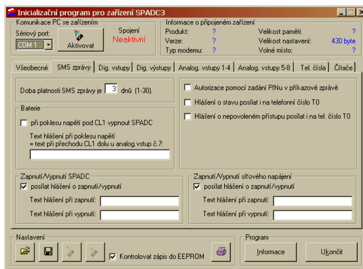
Obrázek 12 – Program SPADC3 Init
